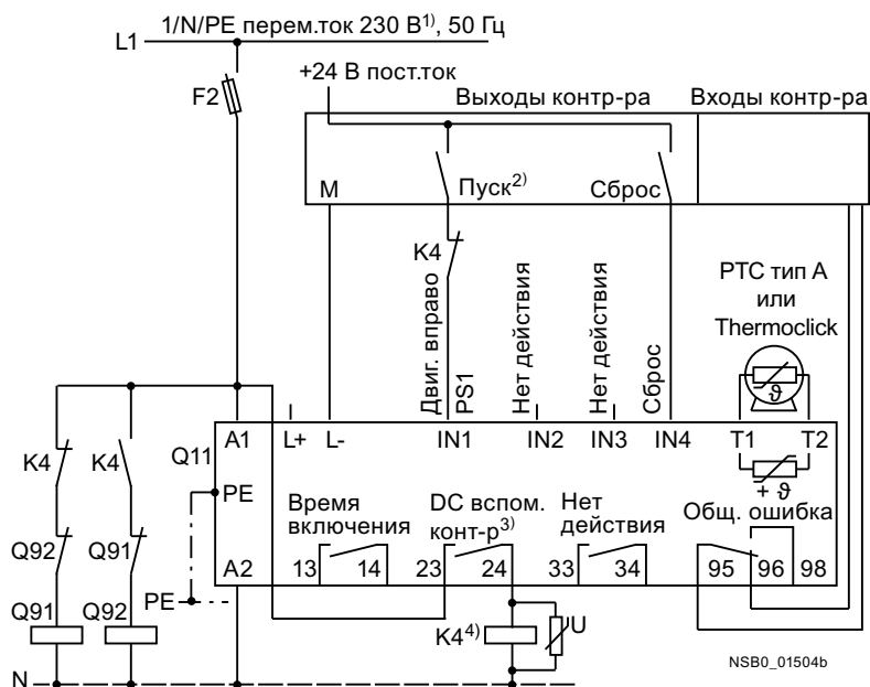
Управляющая электрическая цепь
