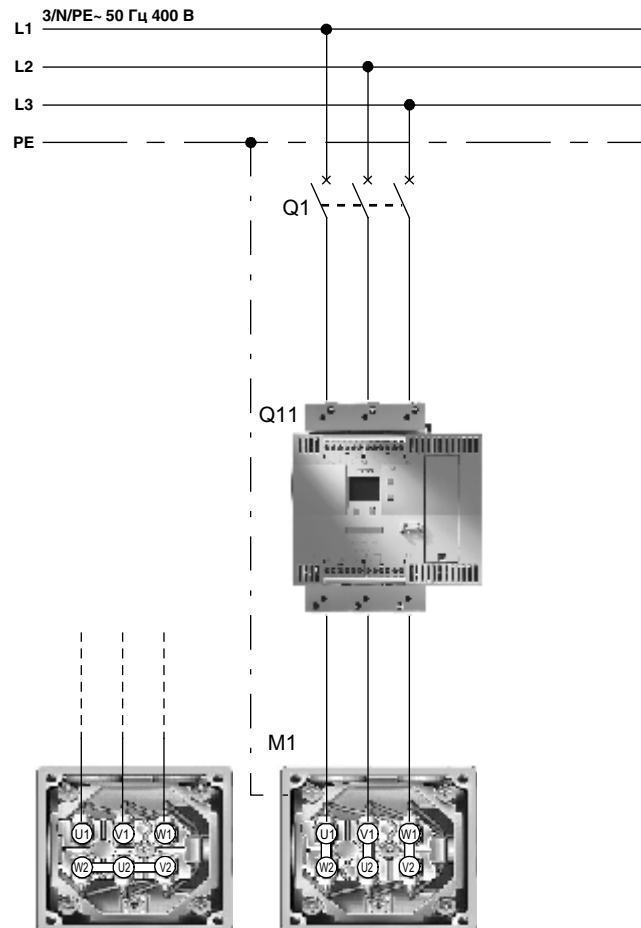
Рисунок 3-3: Принципиальная электрическая схема УПП 3RW44 со стандартным подключением
