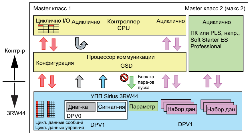
Рисунок 8-2: Принцип коммуникации
