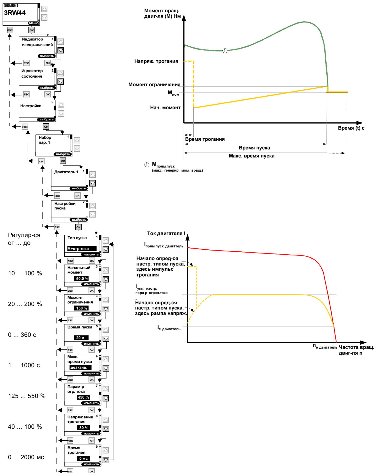
Рисунок 5-11: Тип пуска "Рег. вращ. мом. с ограничением тока"
