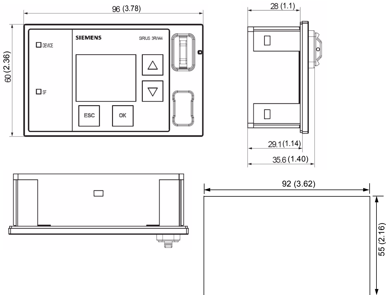
Размеры в мм (дюймах)
