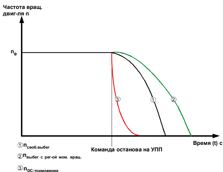
Рисунок 6-6: Типы выбега, общая информация
